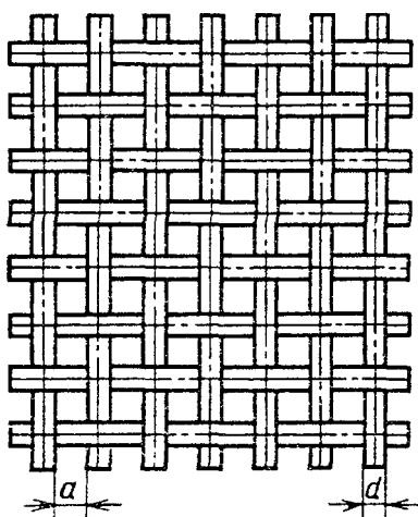
Плотняное переплетение
