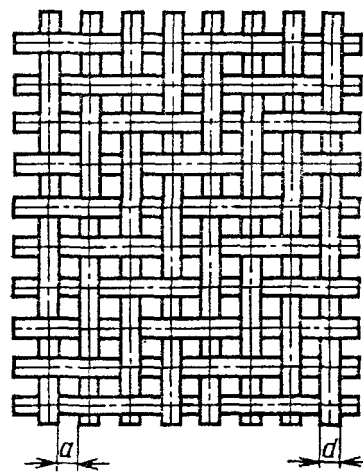
Саржевое переплетение
